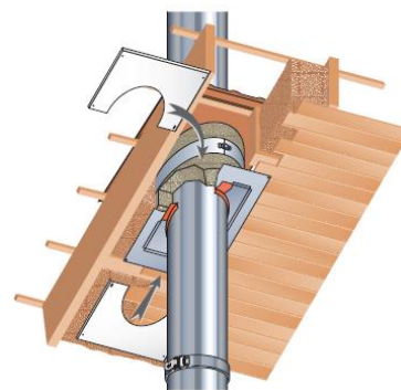
SOLUTION PLAFOND RAMPANT
